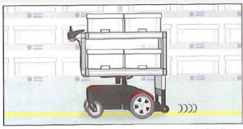
簡単に敷設できる反射テープのラインを検出
