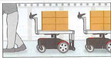
レーザーセンサーで追従対象を区別
