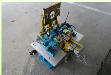
溶接設備で使用する特注治具
