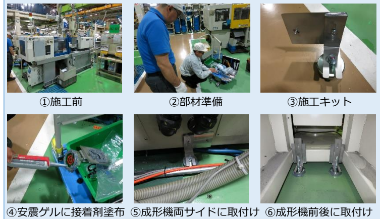
① 施工前 ② 部材準備 ③ 施工キット ④ 安震ゲルに接着剤塗布 ⑤ 成形機両サイドに取付け ⑥ 成形機前後に取付け
