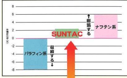
ゴム膨潤試験結果(部材:NBR 試験条件:150℃×70h) 自社調べ
